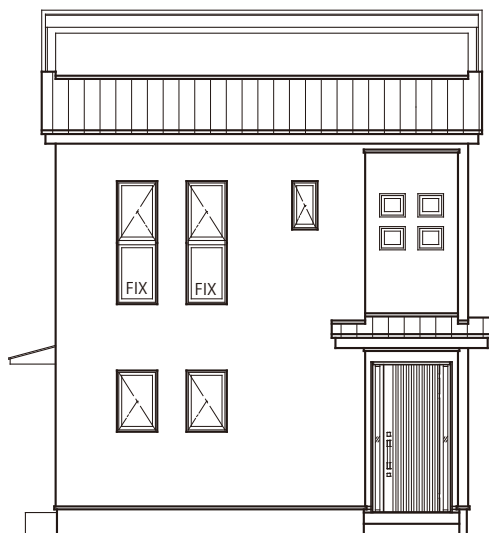
北面 立面图
