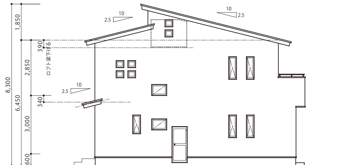
西面 立面图
