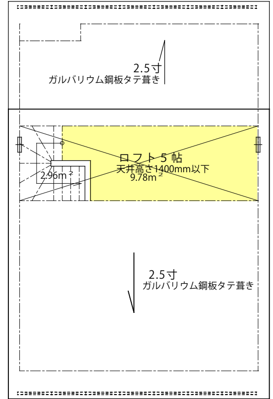
屋根平面図
