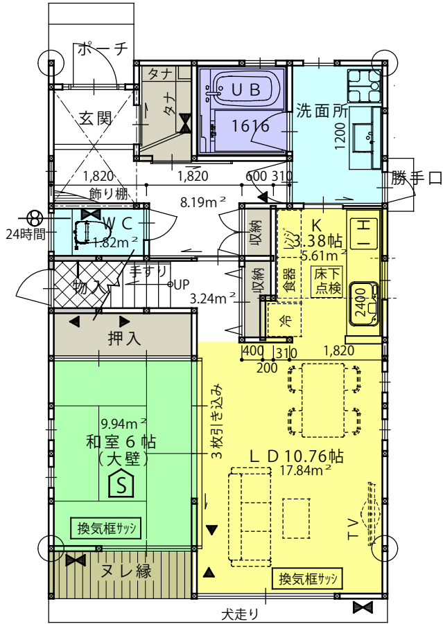
1階平面図
