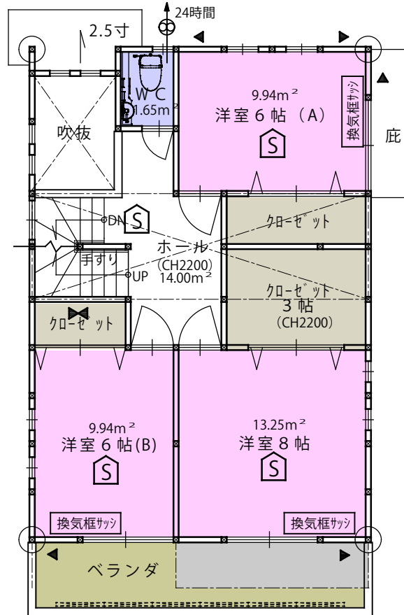
2階平面図
